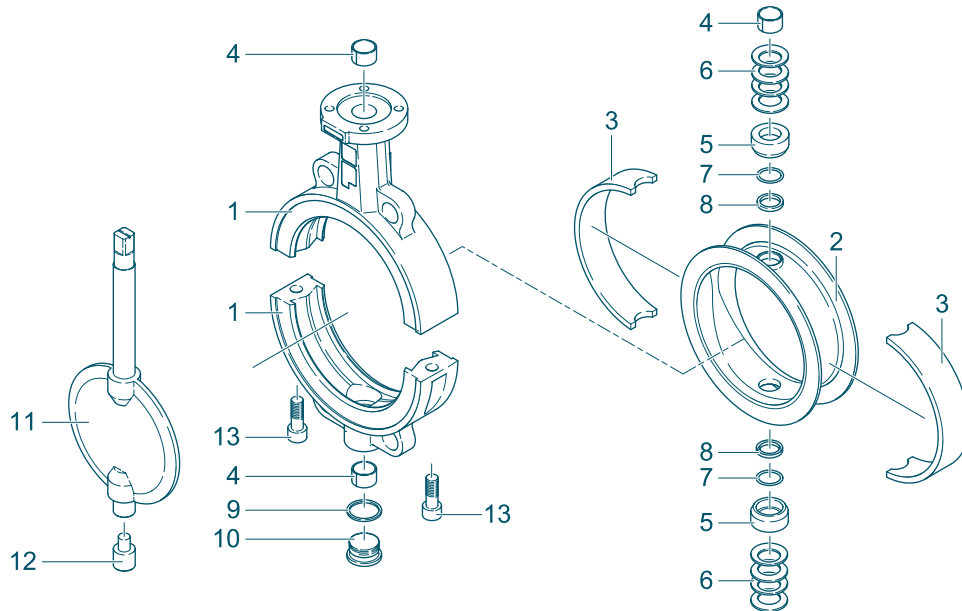
Межфланцевый затвор с уплотнением PTFE DN 80-200
