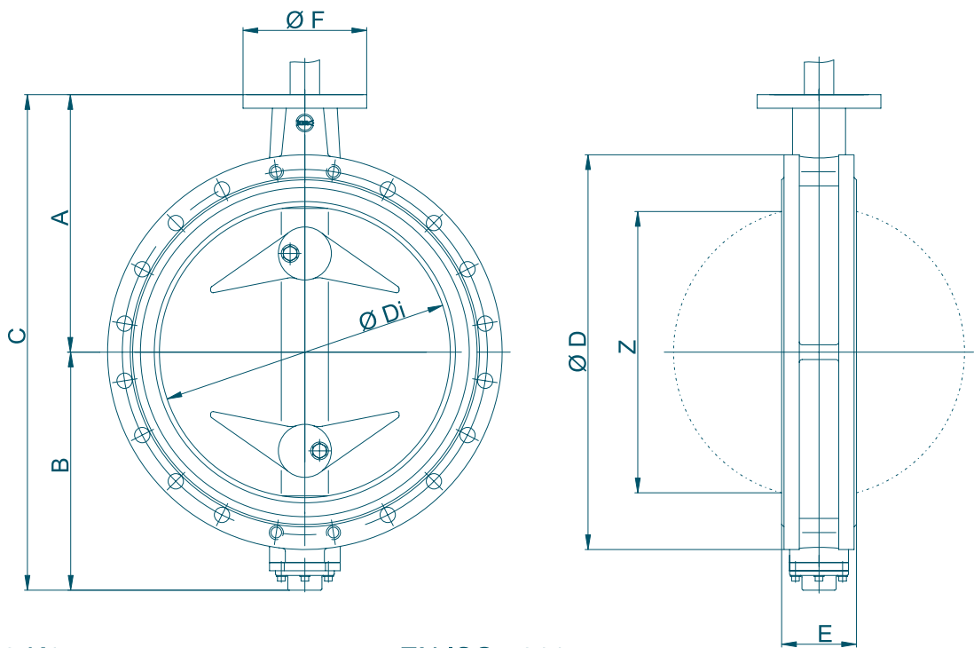
F012-K1 с голым валом согласно EN ISO 5211
