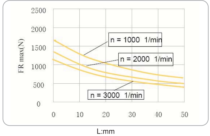
FO=200N
