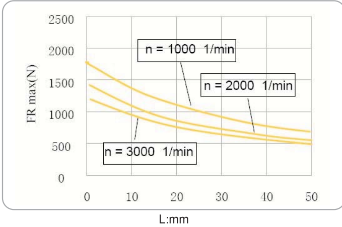
FO=0N
